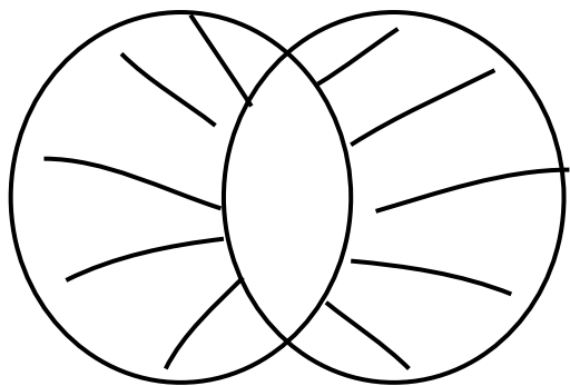
симметрическая разность
